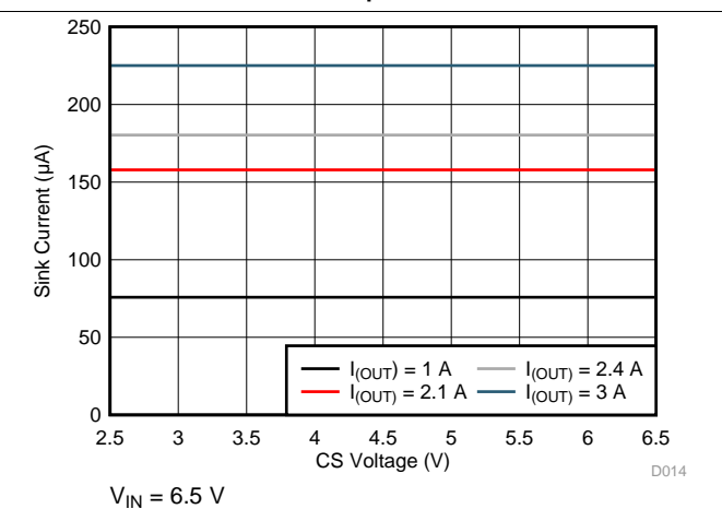
Figure 14. I_{CS} vs V_{CS} Voltage
